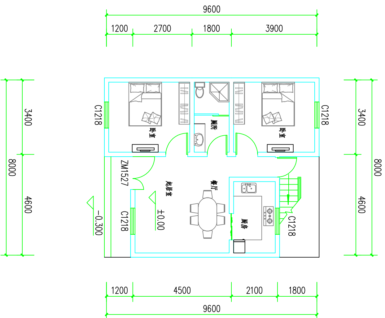
一层平面图
